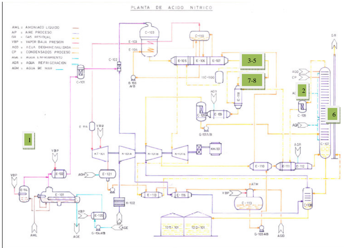
Ilustración: Diagrama de flujo de la planta de ácido nítrico Fertiberia Sagunto.
